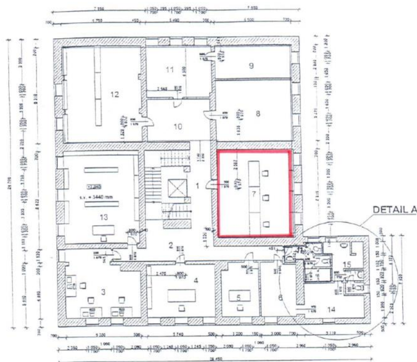
PŮDORYS 2.NP M 1:150
